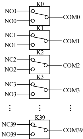
图 2-2-1 硬件框图
