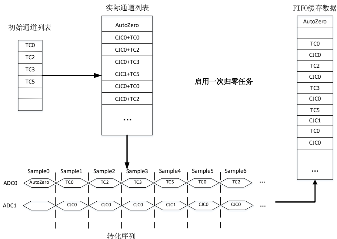
图 4-4-3 一次归零
