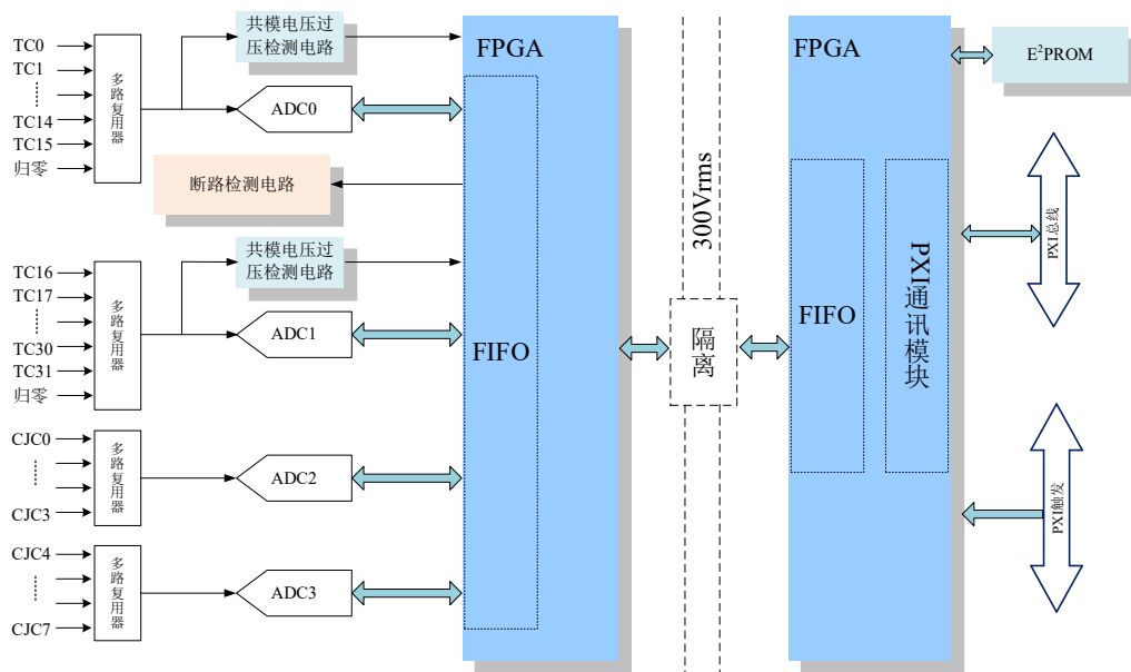
图 2-2-2 PXI8092 系统框图
