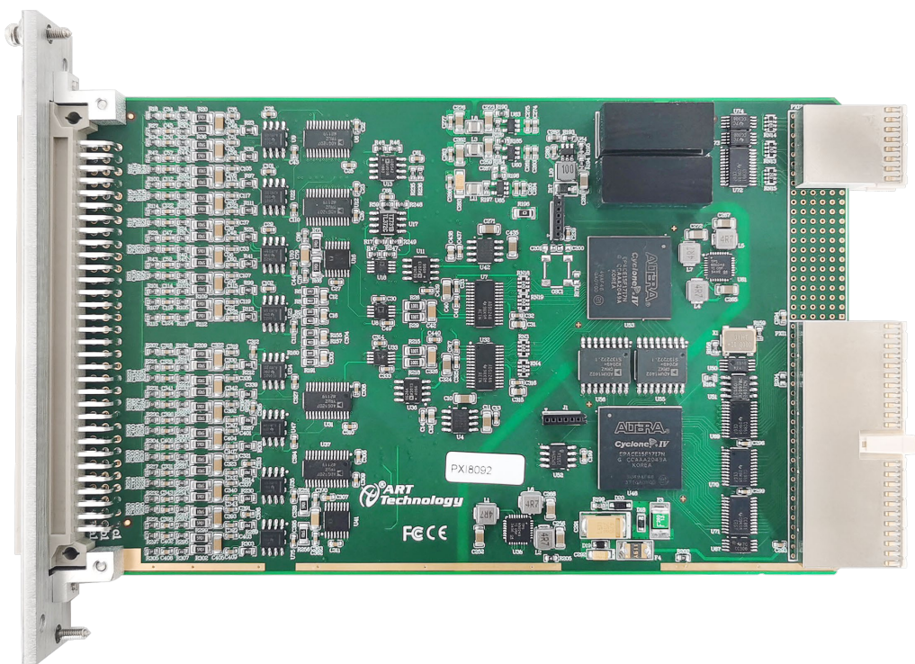
图 3-1-2 PXI8092 外形图
