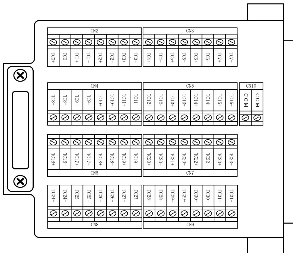
图 3-3-2 TB8092 端子引脚定义
