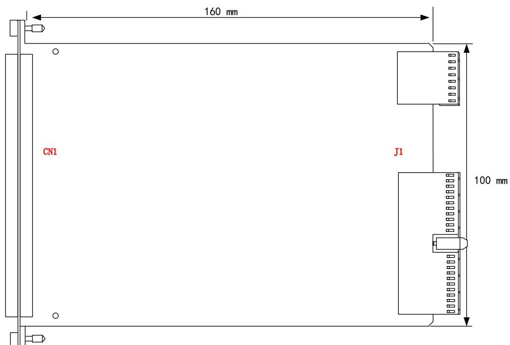
图 3-2-1 PXI890x 板卡尺寸图
