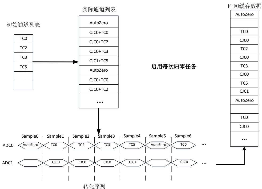
图 4-4-2 每次归零
