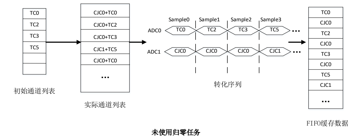
图 4-4-1 不启动归零
