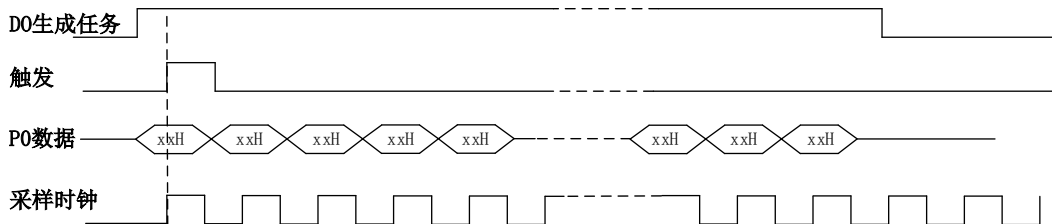
图7-7-3 内、外时钟连续生成
