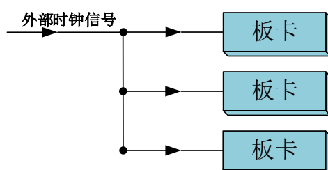
图4-9-4 外时钟同步采集的连接方式
