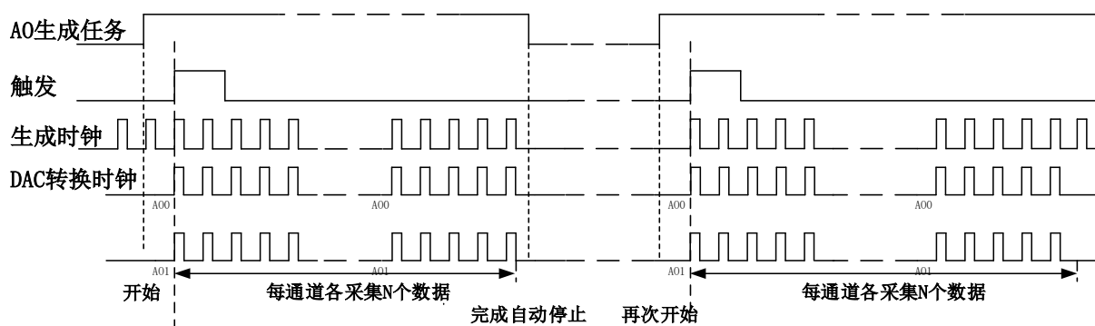
图5-7-2 内、外时钟有限点生成
