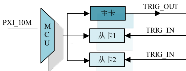
图 4-9-1 采用工控机箱背板的 PXI_10M 时钟信号作为时钟参考源
