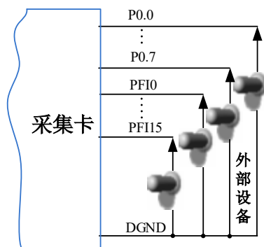
图7-3-1 DI 数字量输入的连接
