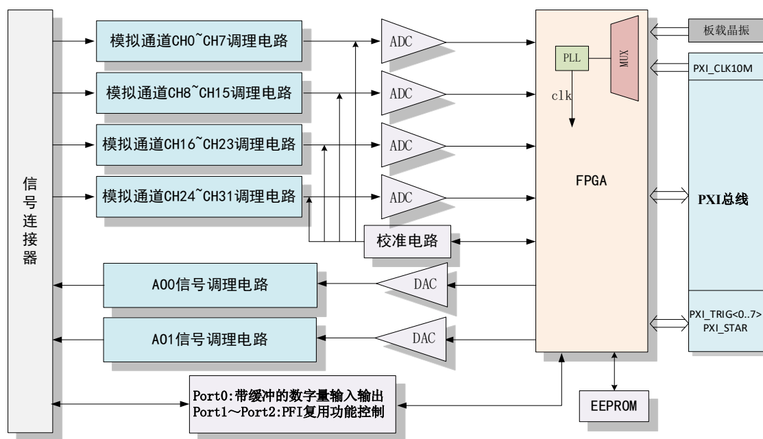
图2-2-1 PXI9774 系统框图
