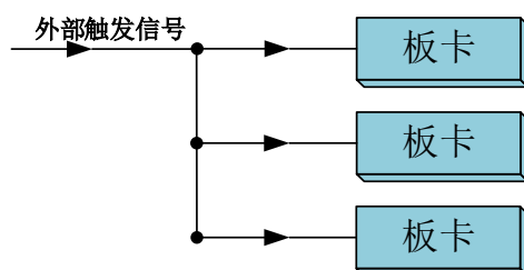
图 4-9-3 外触发同步采集的连接方式
