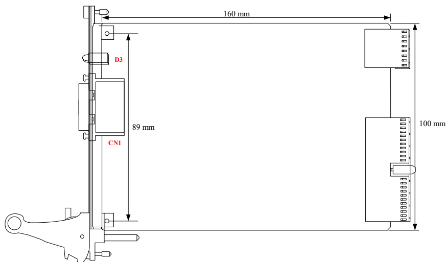
图 3-1-1 PXI9774 板卡尺寸图
