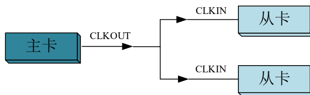
图 4-9-2 主从卡时钟级联同步采集的连接方式
