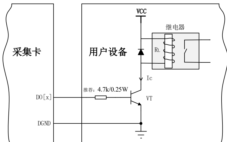
图 7-4-2 DO 数字量控制继电器电路
