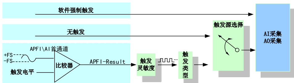
图 8-1-2 模拟触发源选择
