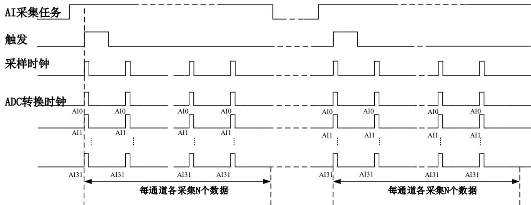
图 4-7-2 有限点采样
