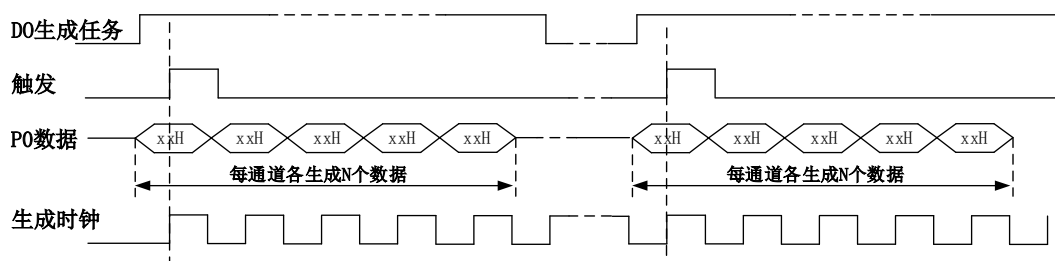
图7-7-2 有限点生成
