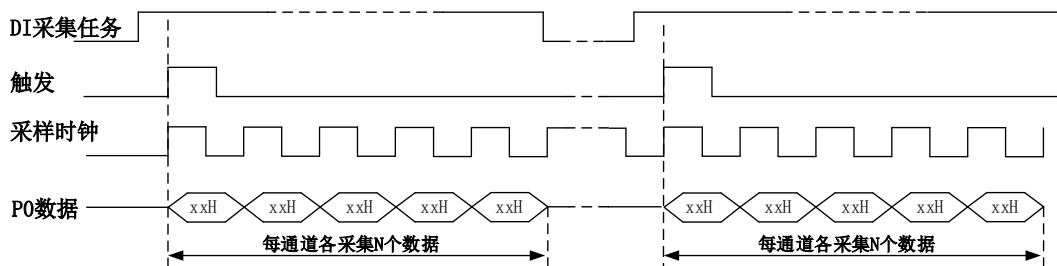
图 7-6-2 有限点采样
