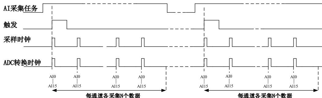
图 4-7-2 有限点采样
