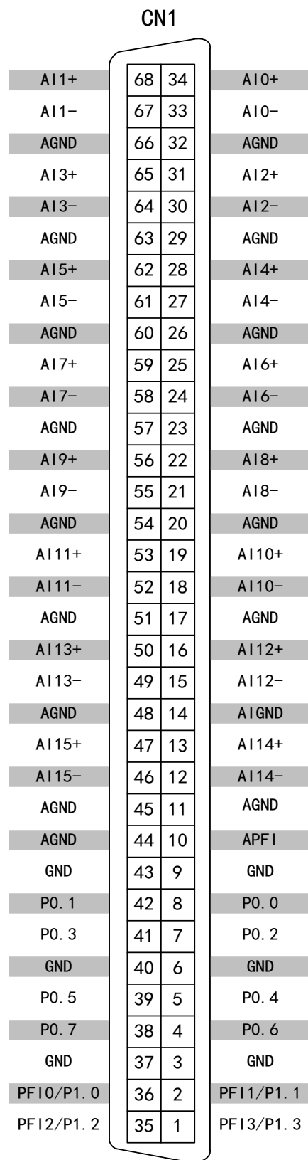
图 3-3-1 PXI9009\A\B 管脚定义图
