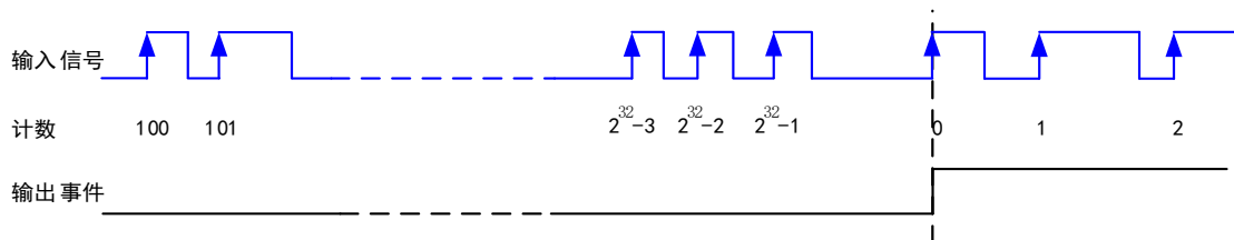
图 5-10-2 反转方式输出
