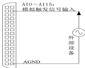
图7-3-3 模拟触发连接方法
