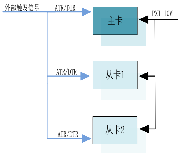
图 4-9-2 共同的外触发信号
