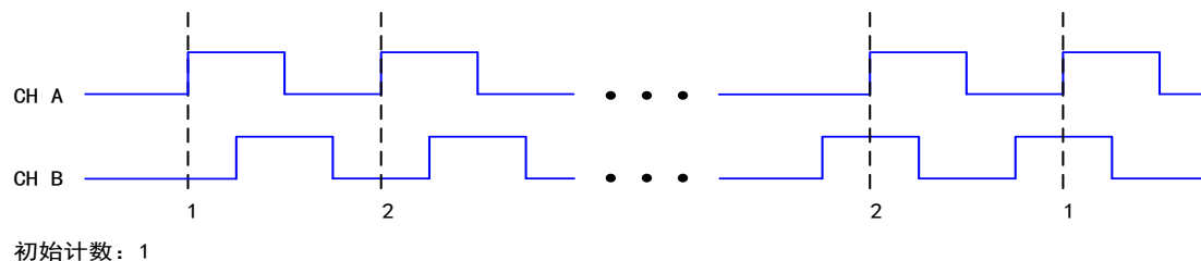
图 5-7-1 X1 编码
