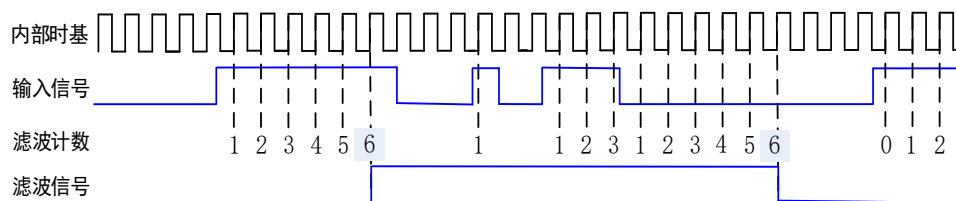
图 5-9-1 脉冲输出
