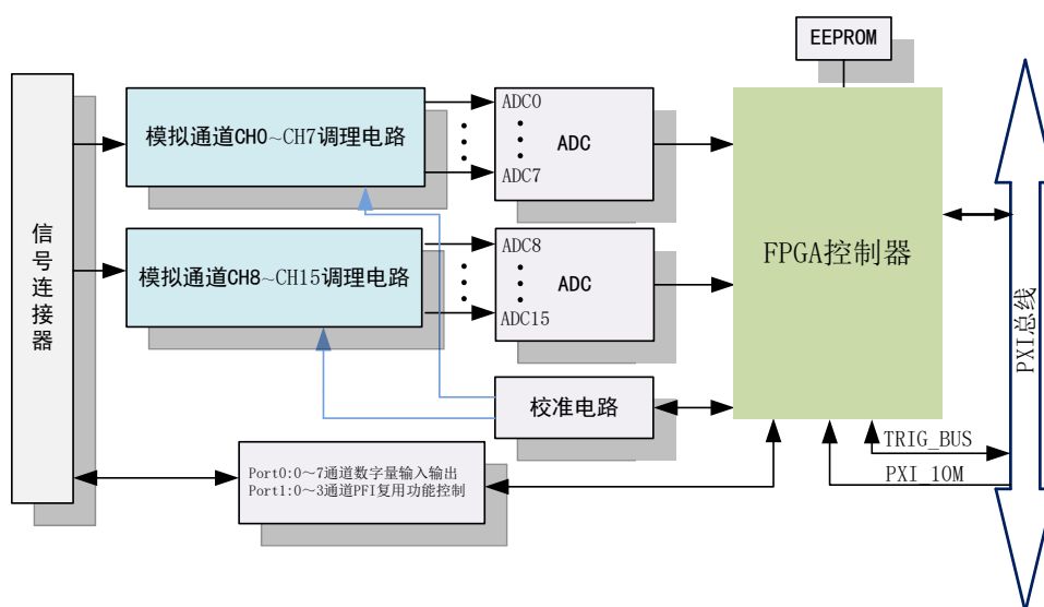
图 2-2-1 PXI9009\A\B 系统框图
