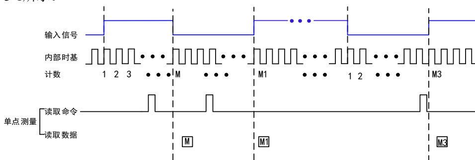
图 5-3-1 半周期示意图
