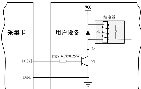
图 6-3-1 DO 数字量控制继电器电路
