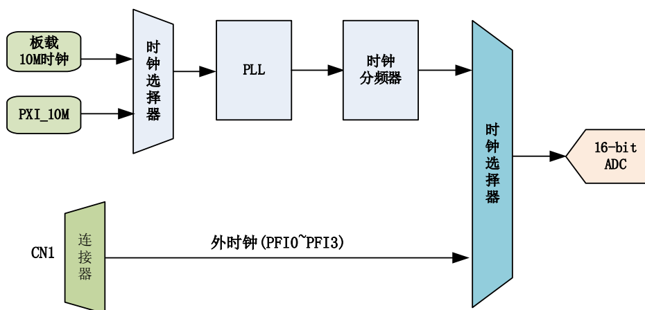
图 4-6-1 AI 时钟结构框图
