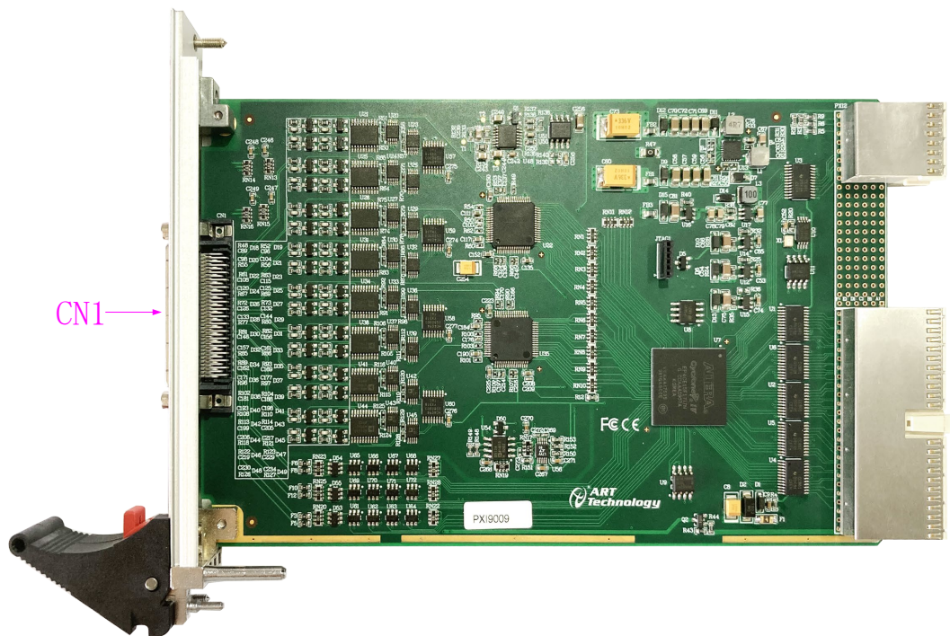
图 3-1-1 PXI9009\A\B 板卡外形图
