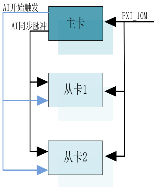
图 4-9-1 主从卡级联
