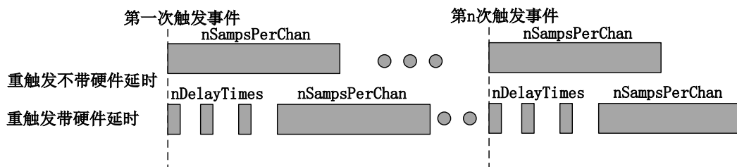
图 7-2-5 AI 重触发
