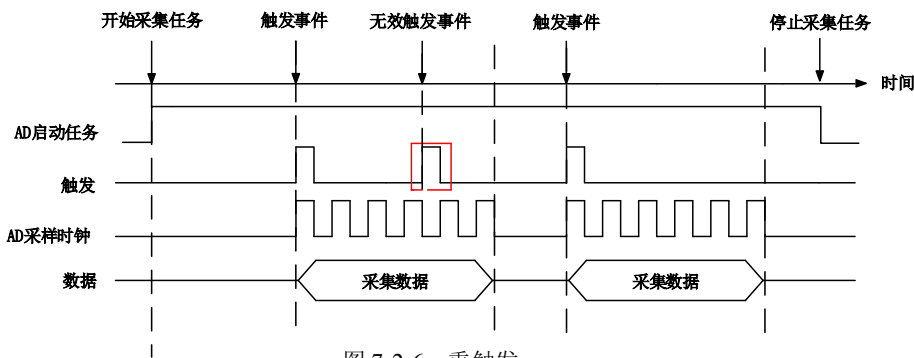
图 7-2-6 重触发
