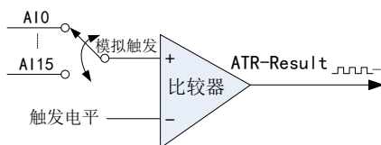
图7-3-4 模拟触发比较器
