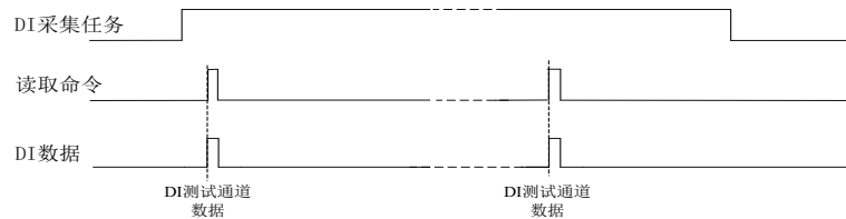
图6-5-1 按需单点采集
