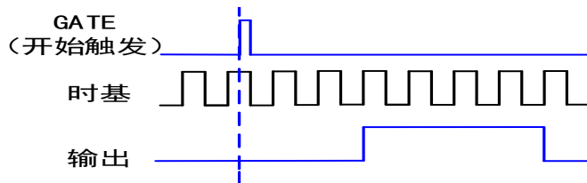
图 5-8-2 具有启动触发的单脉冲生成
