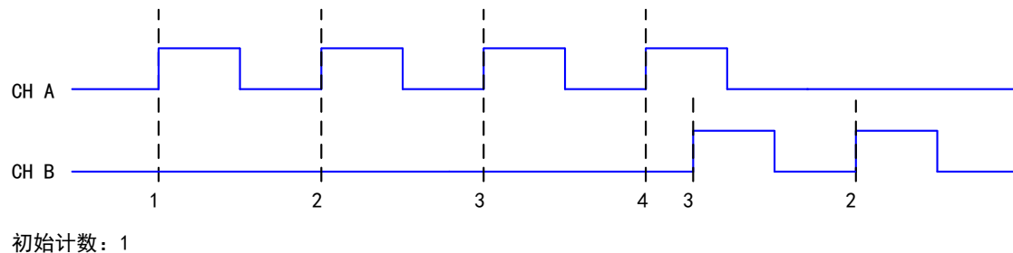
图 5-7-4 双脉冲编码
