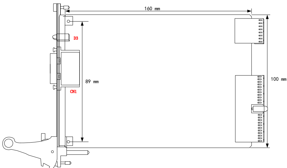
图 3-2-1 PXI9009\A\B 板卡尺寸图
