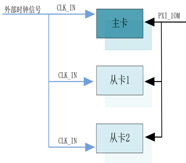
图 4-9-3 共同的外时钟信号
