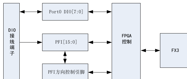
图6-1-1 DIO功能框图
