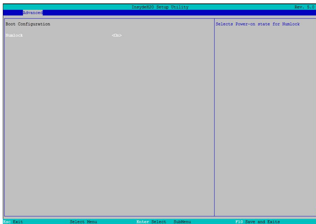
图 6 Numlock 配置
