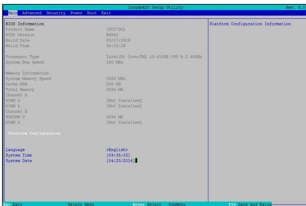
图 3 主界面信息
