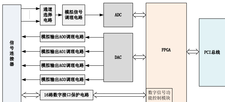
图2-2-1 PCI5640/1/2/3 系统框图
