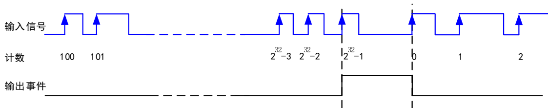
图 6-10-1 脉冲方式输出
