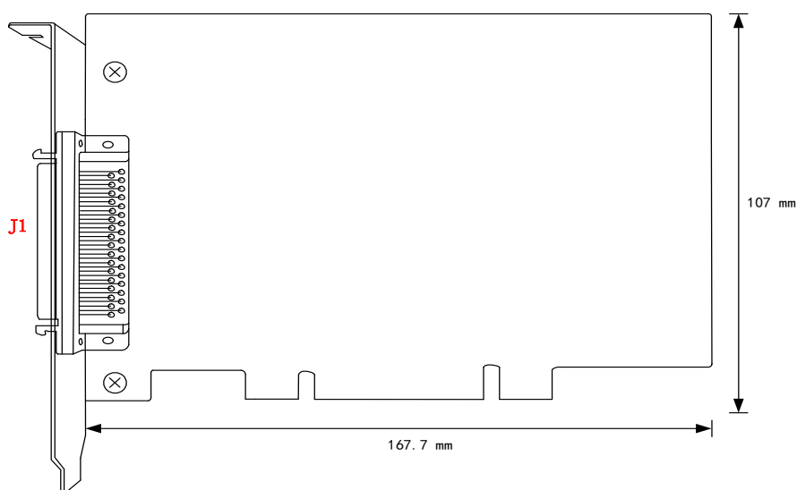
图 3-2-1 外壳尺寸图
