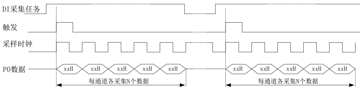
图 7-5-2 有限点采样
