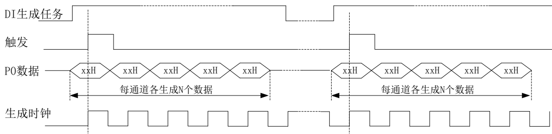
图7-6-2 有限点生成
