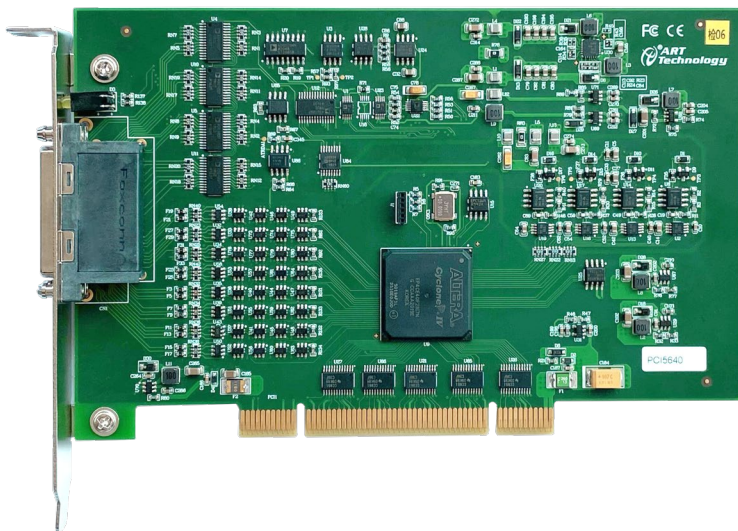
图 3-1-1 PCI5640/1/2/3 正面图
